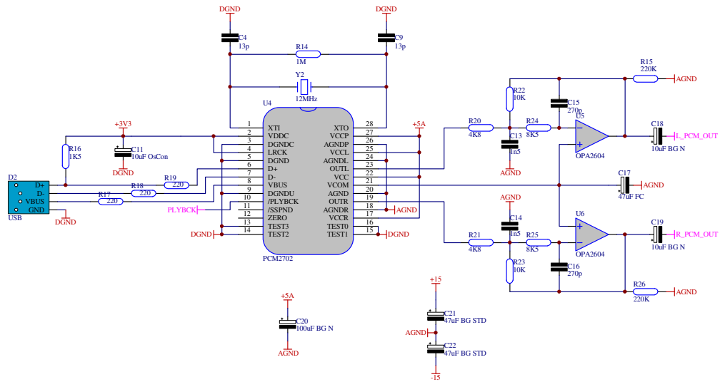
PCM2702 USB DAC Krzysztof Marcinek kafka85@o2.pl
